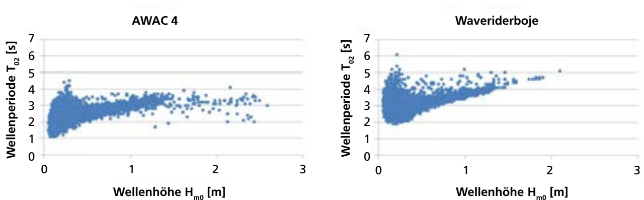
1.11 > Messergebnisse mit Hinblick auf Wellenhöhe und -periode von AWAC 4 und der Waveriderboje
