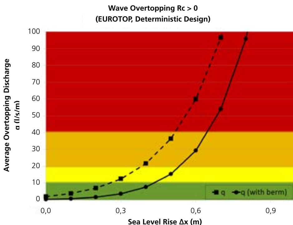
1.5 > Mittlere Wellenüberlaufmengen bei einfach geneigtem Deich sowie Deich mit Berme in Abhängigkeit vom Meeresspiegelanstieg
