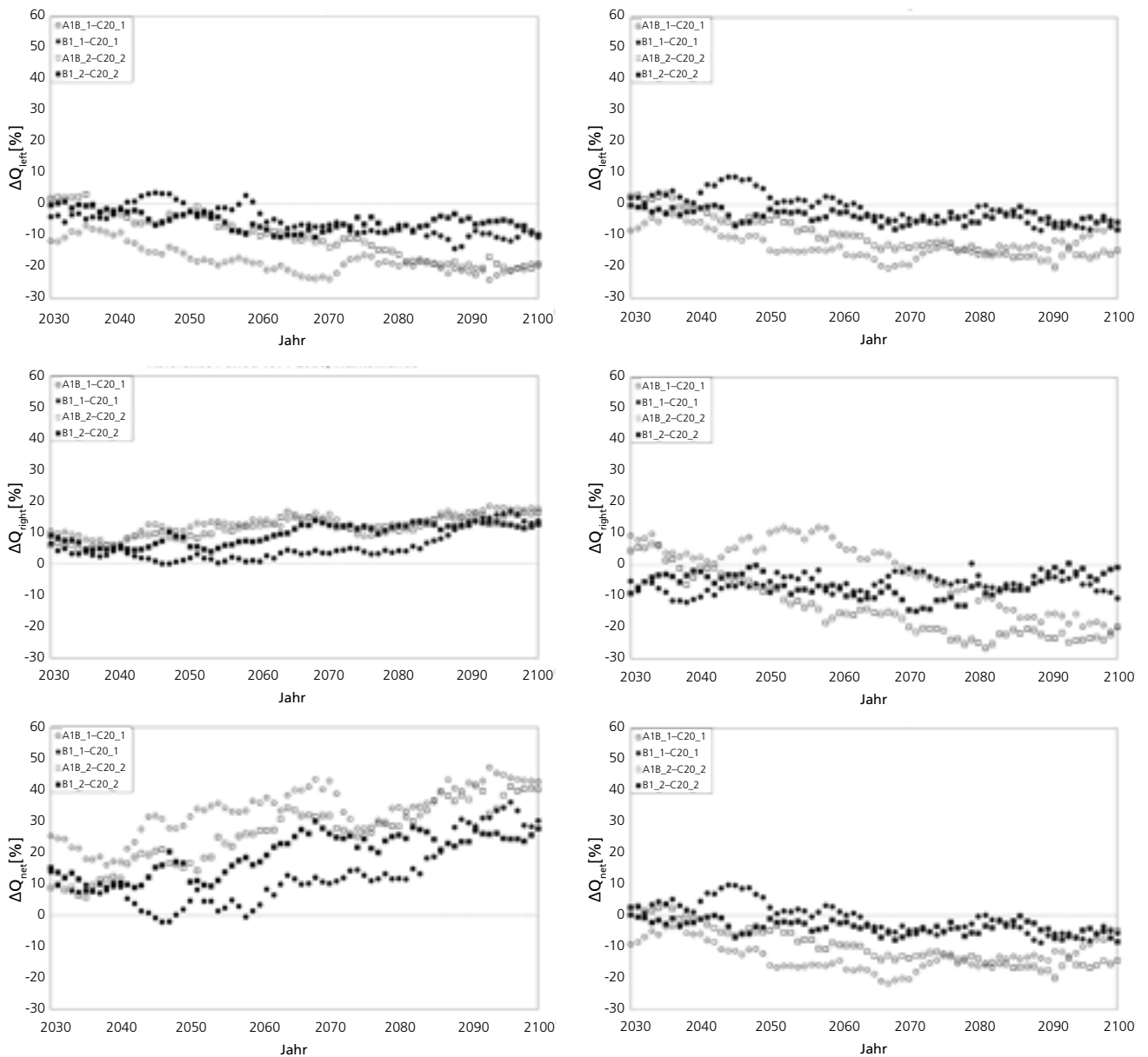
2.15 > Veränderung der gerichteten ( \Delta Q_{\text{left}} , oben bzw. \Delta Q_{\text{right}} , mittig) und Netto-Sedimenttransportkapazitäten ( \Delta Q_{\text{net}} , unten) über Zeitabschnitte von 30 Jahren, für die Emissionsszenarien A1B und B1, bezogen auf den Referenzzeitraum C20 (1971–2000) in der Nähe von Warnemünde (links) und Timmendorfer Strand (rechts)
