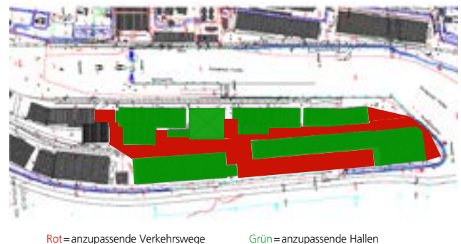
1.62 > Notwendige Anpassungsbereiche bei 20 cm Meeresspiegelanstieg
